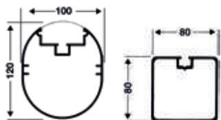
POSTE Y LARGUERO
