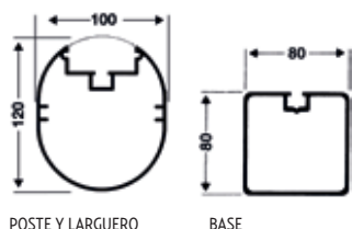
POSTE Y LARGUERO
